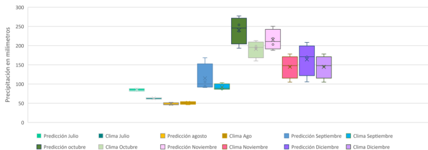
Figura 15. Proyección semestral de la precipitación por mes en la zona Sur y Guachinte
