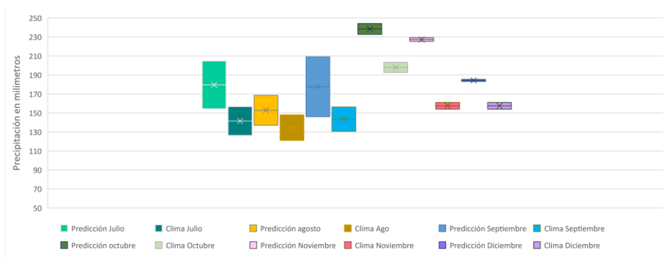
Figura 9. Proyección semestral de la precipitación por mes en el valle del río Risaralda
