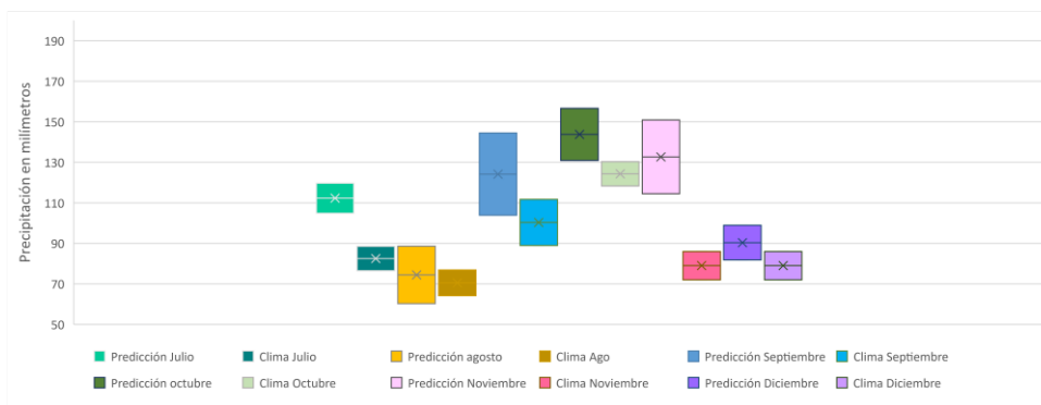
Figura 10. Proyección semestral de la precipitación por mes en la zona Norte 2a
