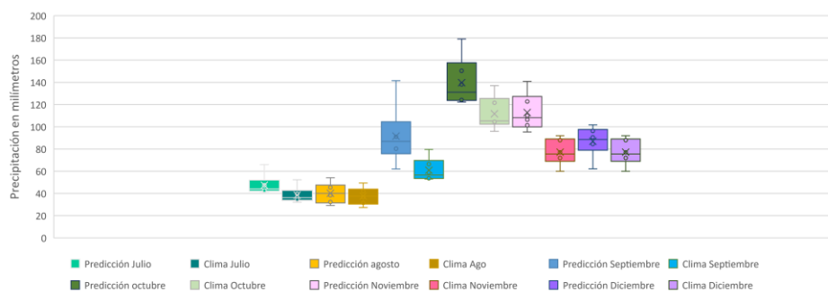
Figura 12. Proyección semestral de la precipitación por mes en la zona Centro Occidente
