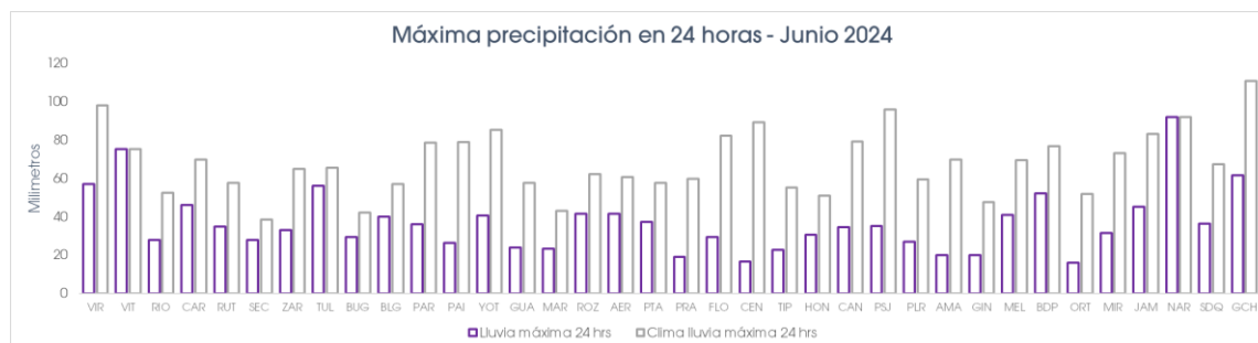
Figura 4a. Máxima precipitación en milímetros en 24 horas en junio de 2024
