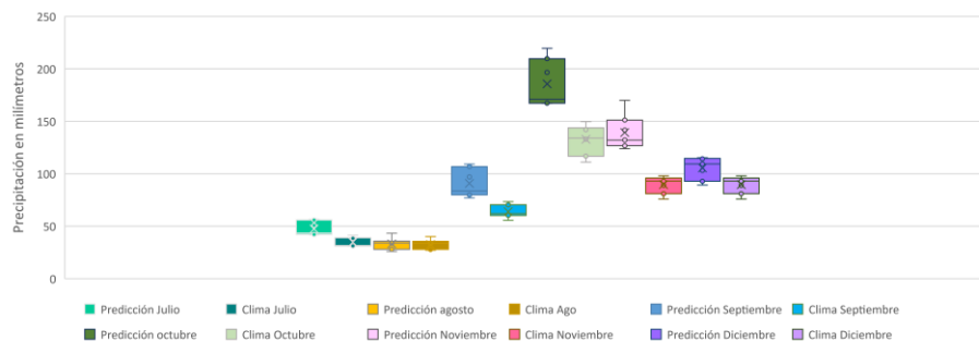
Figura 13. Proyección semestral de la precipitación por mes en la zona Centro Oriente
