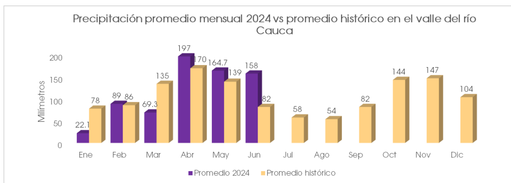
Figura 1. Precipitación promedio en junio y promedio climatológico en el VRC
