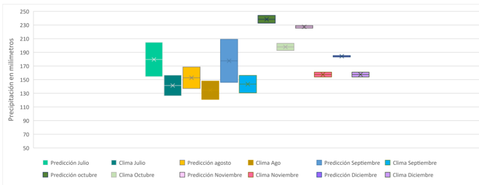
Figura 11. Proyección semestral de la precipitación por mes en la zona Norte 2b
