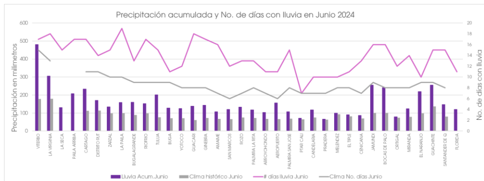
Figura 3. Valores de lluvia acumulada en junio y número de días según la red meteorológica de Cenicaña. https://www.cenicana.org/apps/meteportal/public/diarios
