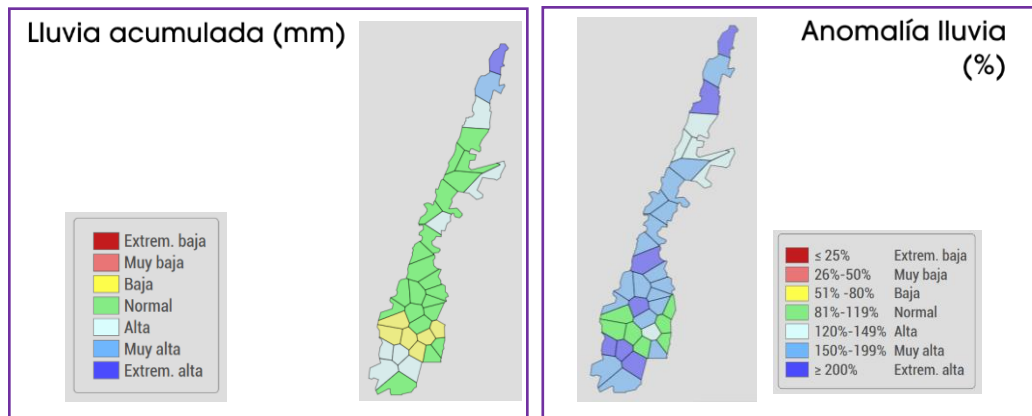
Figura 2. Precipitación acumulada en el mes de junio (izquierda) y su respectiva anomalía (derecha).
