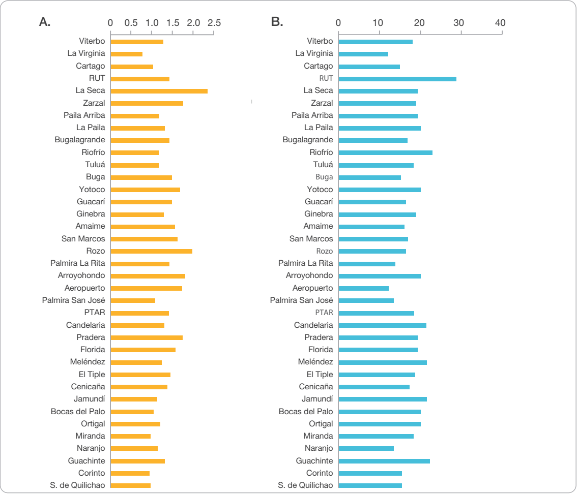
Figura 5. (A) Velocidad media del viento a 10 metros de altura, medida en las estaciones meteorológicas del sector. (B) Máxima velocidad del viento medida en las mismas estaciones.
