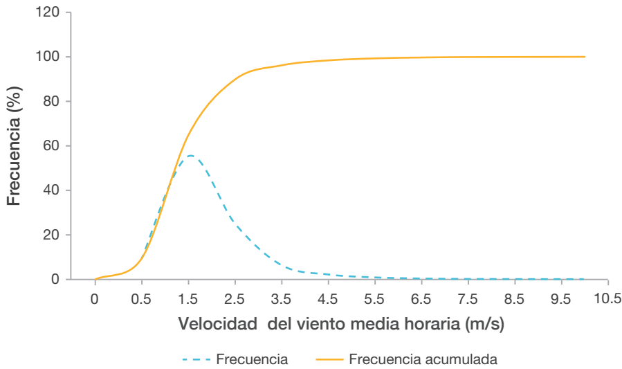
Figura 2. Frecuencia de ocurrencia de diferentes velocidades del viento a escala horaria en el valle del río Cauca (2010-2019).
