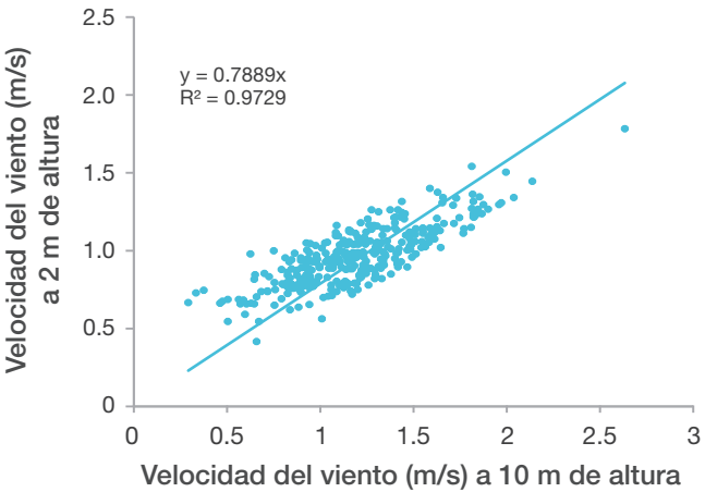
Figura 6. Relación entre la velocidad del viento medida a 10 m y a 2 m de altura sobre la superficie en la estación Cenicaña (Florida, Valle del Cauca).
