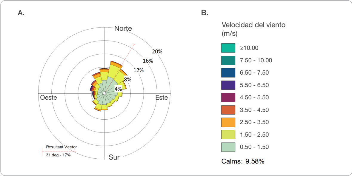
Figura 3. (A) Dirección media del viento, y (B) su velocidad en el valle del río Cauca (periodo de los datos?).
