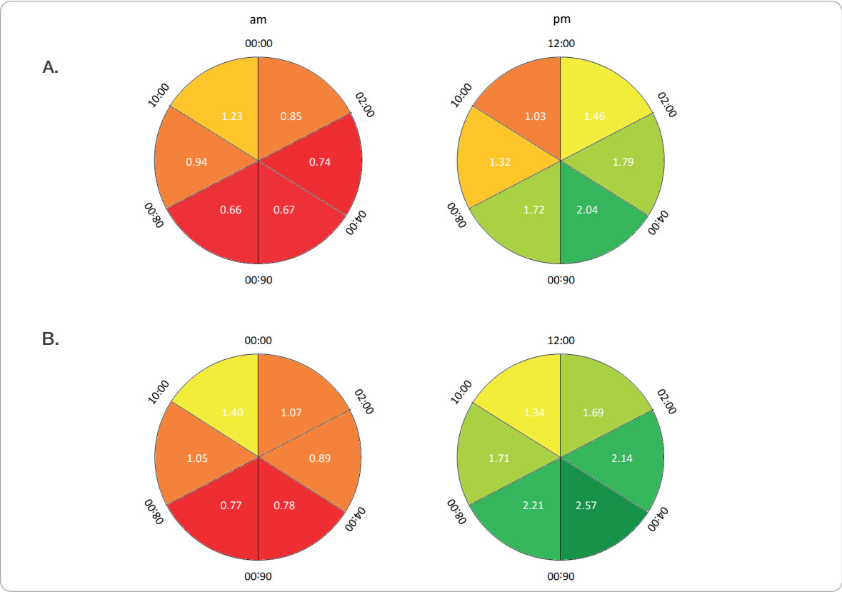
Figura 4. Velocidad media del viento en el valle del río Cauca en diferentes horas del día para dos meses del año: (A) mayo y (B) agosto.
