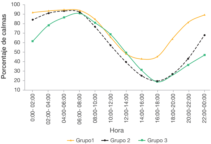
Figura 14. Características de los grupos que describen el comportamiento del porcentaje de horas con velocidad del viento inferior a 1.5 m/s.
